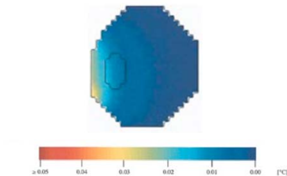
Figure 27 : Simulation de la distribution de l'élévation de la température sur l'œil pour 10 W/m 2 à 30 GHz (Bernardi et al. , 1998)
