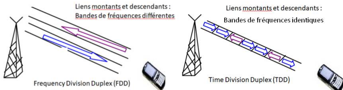
Figure 12 : Principe de fonctionnement de la technique de duplexage FDD et TDD
